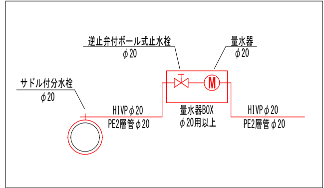
量水器φ20場合（φ30の場合も同様）
