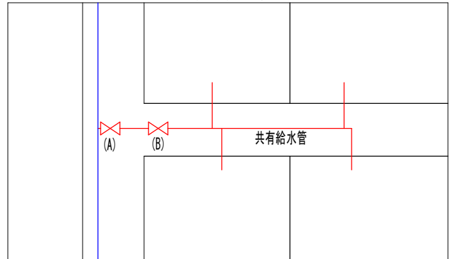
共有給水管設置の場合
