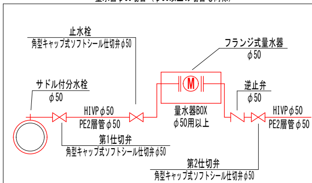
量水器φ50場合（φ50以上の場合も同様）
