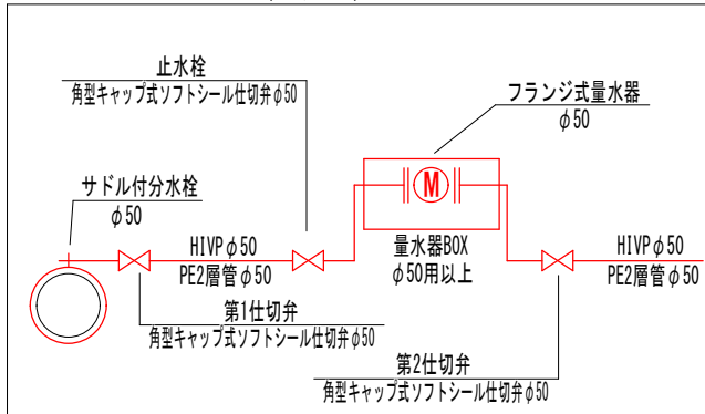
量水器φ50場合（φ50以上も同様）
