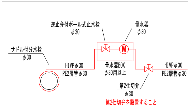
量水器φ30場合（φ40の場合も同様）
