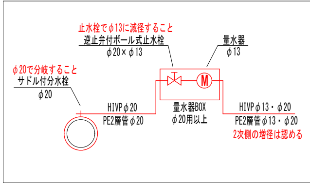
量水器φ13の場合
